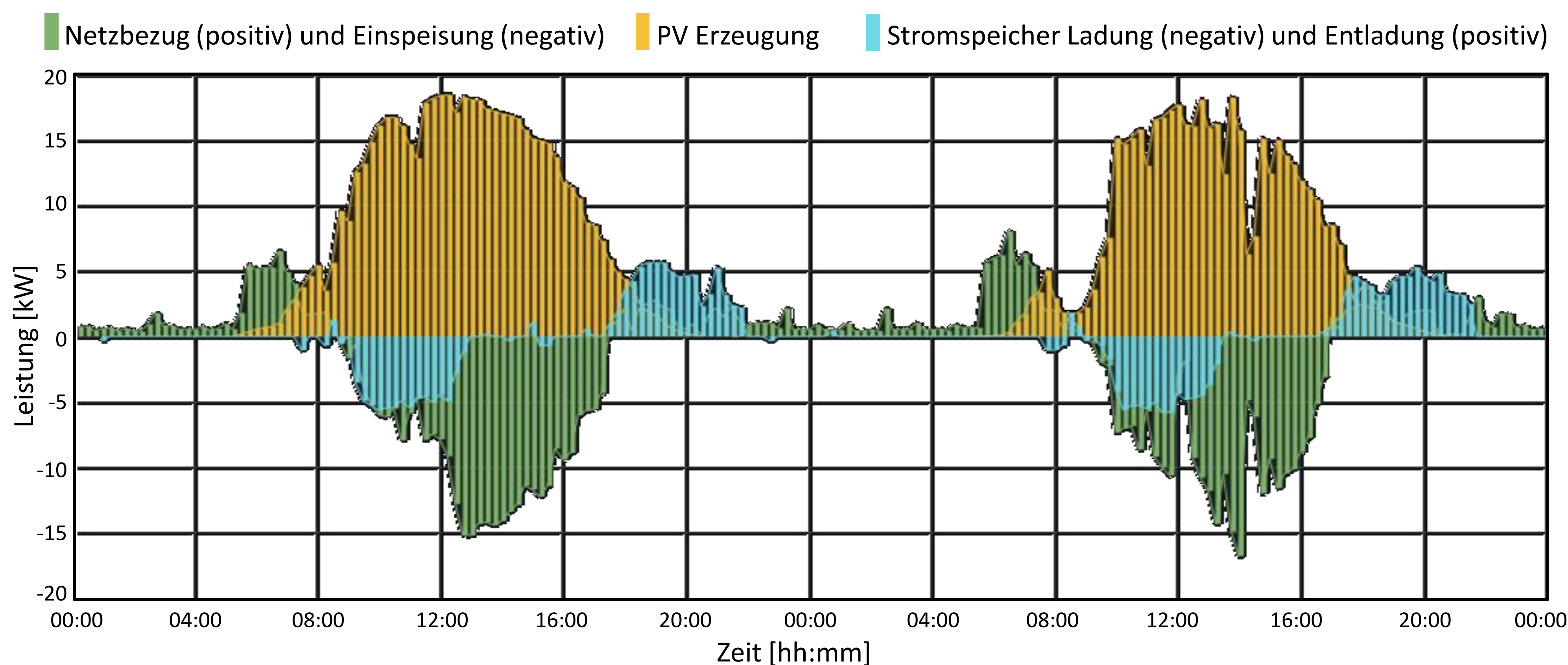
2-Tagesgang Energieflüsse
